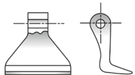
Hammerschlegel Typ „21“
